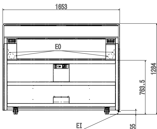
Zij aanzicht
