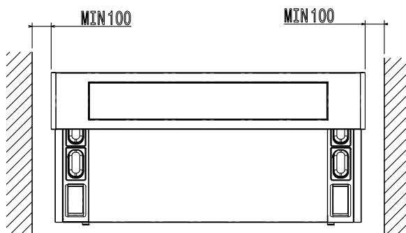
Boven aanzicht
